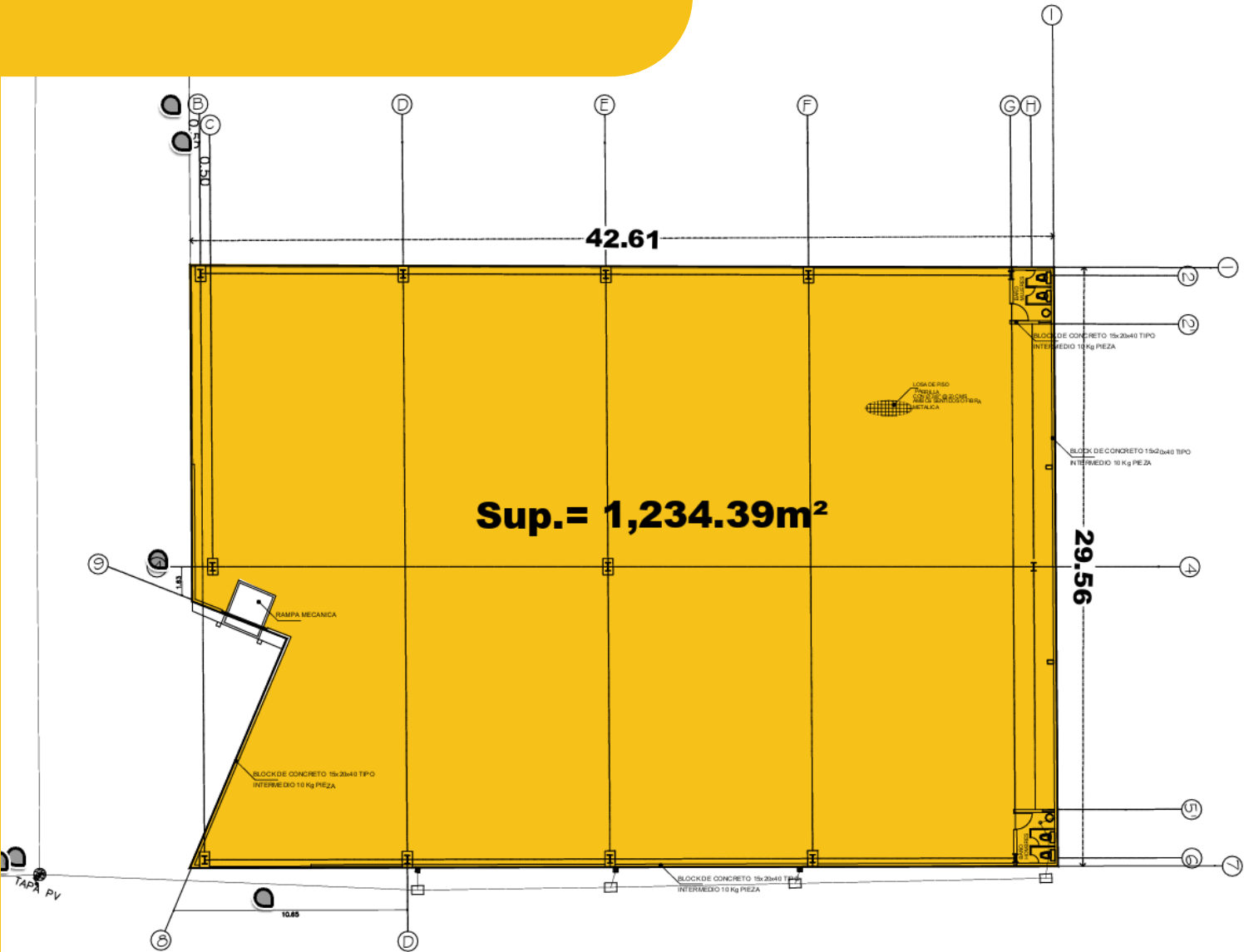
PLANTA ARQUITECTÓNICA BODEGA "E" ARQUITECTÓNICO ESCALA 1:300
