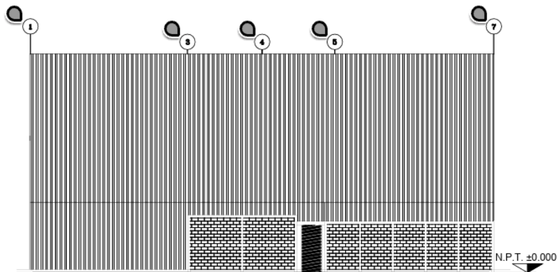
FACHADA PONIENTE ARQUITECTÓNICO
