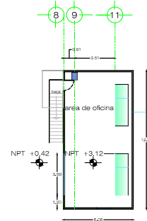
PLANTA ALTA PARA OFICINAS
