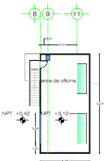
PLANTA ALTA PARA OFICINAS
