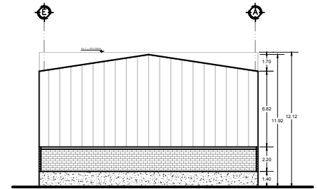
FACHADA TRASERA ESCALA 1:125
