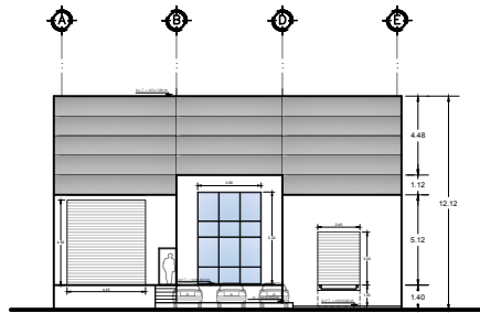
FACHADA FRONTAL ESCALA 1:125
