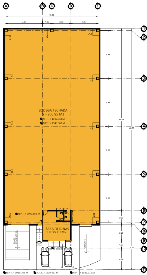
PLANTA ARQUITECTÓNICA ESCALA 1:125
